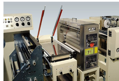
クリーニング装置&つなぎ合せ台
